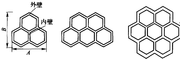
图 6 蜂窝式塑料管横断面形式
