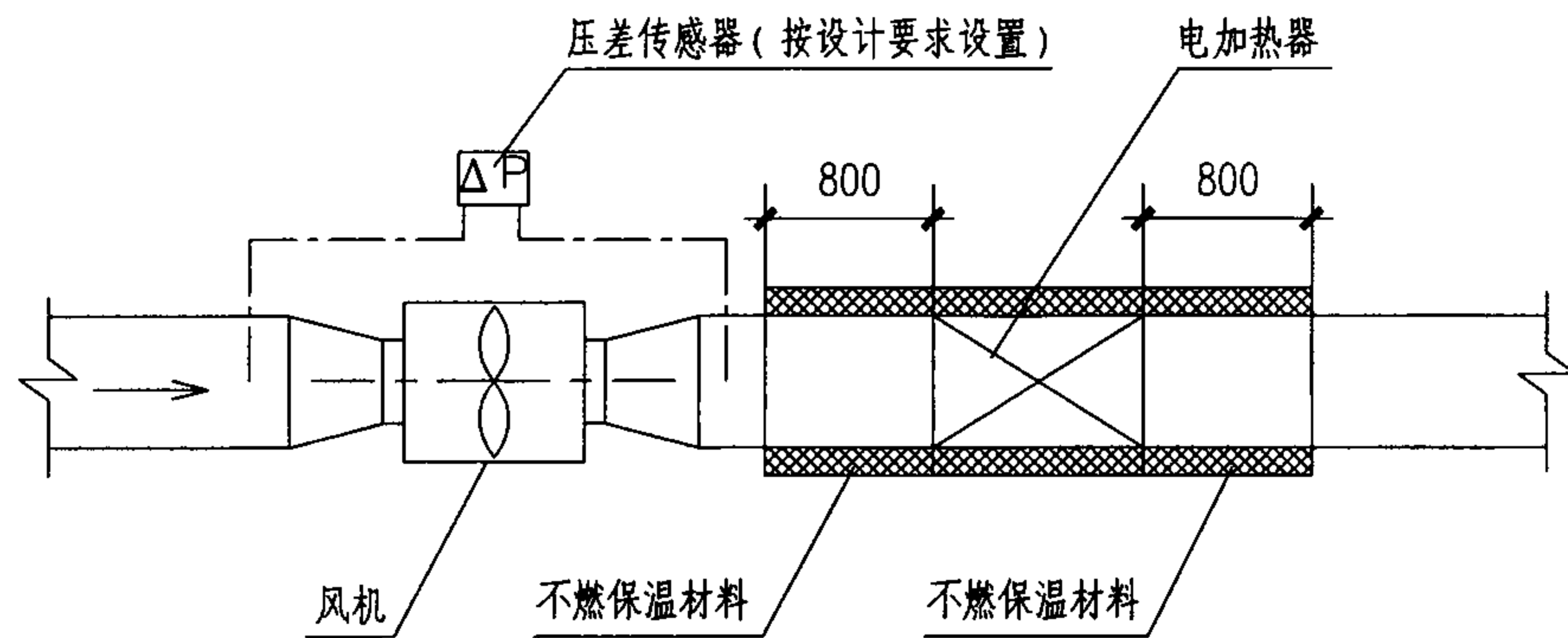
电加热器安装示意图
