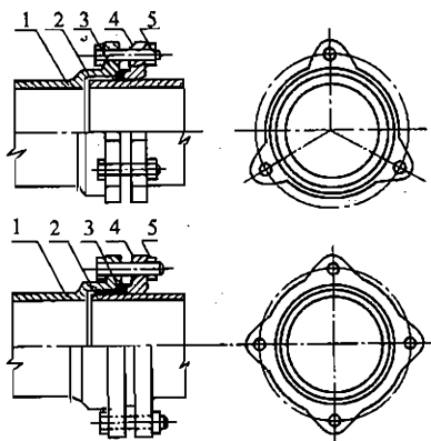
图2 铸铁管法兰机械式接口连接示意图
