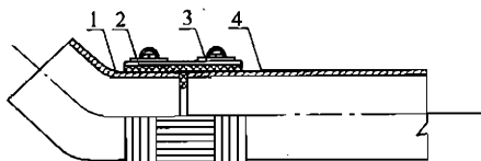
图1 铸铁管卡箍式接口连接示意图
