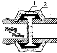
图3 钢管沟槽式连接示意图
